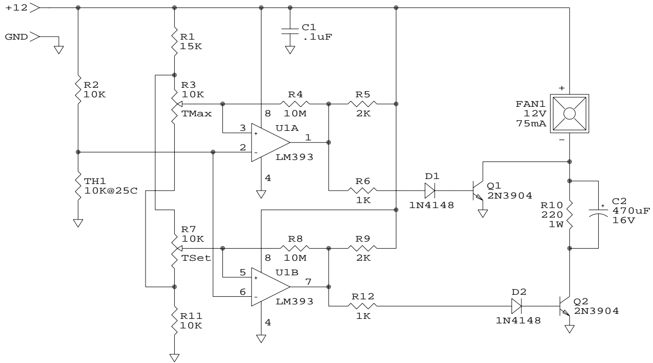
Simple Fan Controller 1
